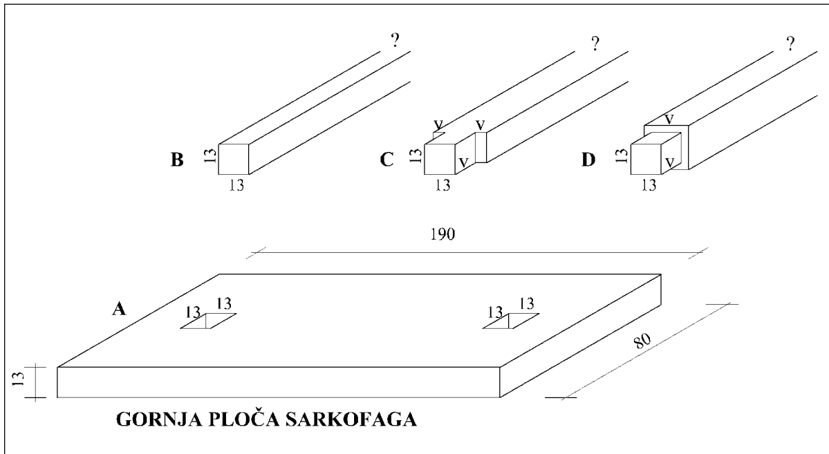
Sl. 10. Tešanj. Ferhad-begov mezar. Hipotetičke varijacije nišana i njihovog uglavljivanja (usađivanja) u gornju ploču sarkofaga. © M. H. Čeman
