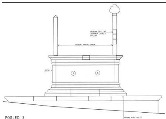
Sl. 6. Tešanj. Ferhad-begov mezar. Crtež rađen s pogledom iz ulice. © Zavod za zaštitu spomenika u sastavu Federalnog ministarstva kulture i sporta / sporta, Sarajevo. Linija terena koja se na crtežu spušta slijeva nadesno pogrešno je ucrtana. Teren pada s desna ulijevo što je jasno vidljivo iz ulice iz koje su promatrane potkonstrukcija i sarkofag koji su prikazani na crtežu.
